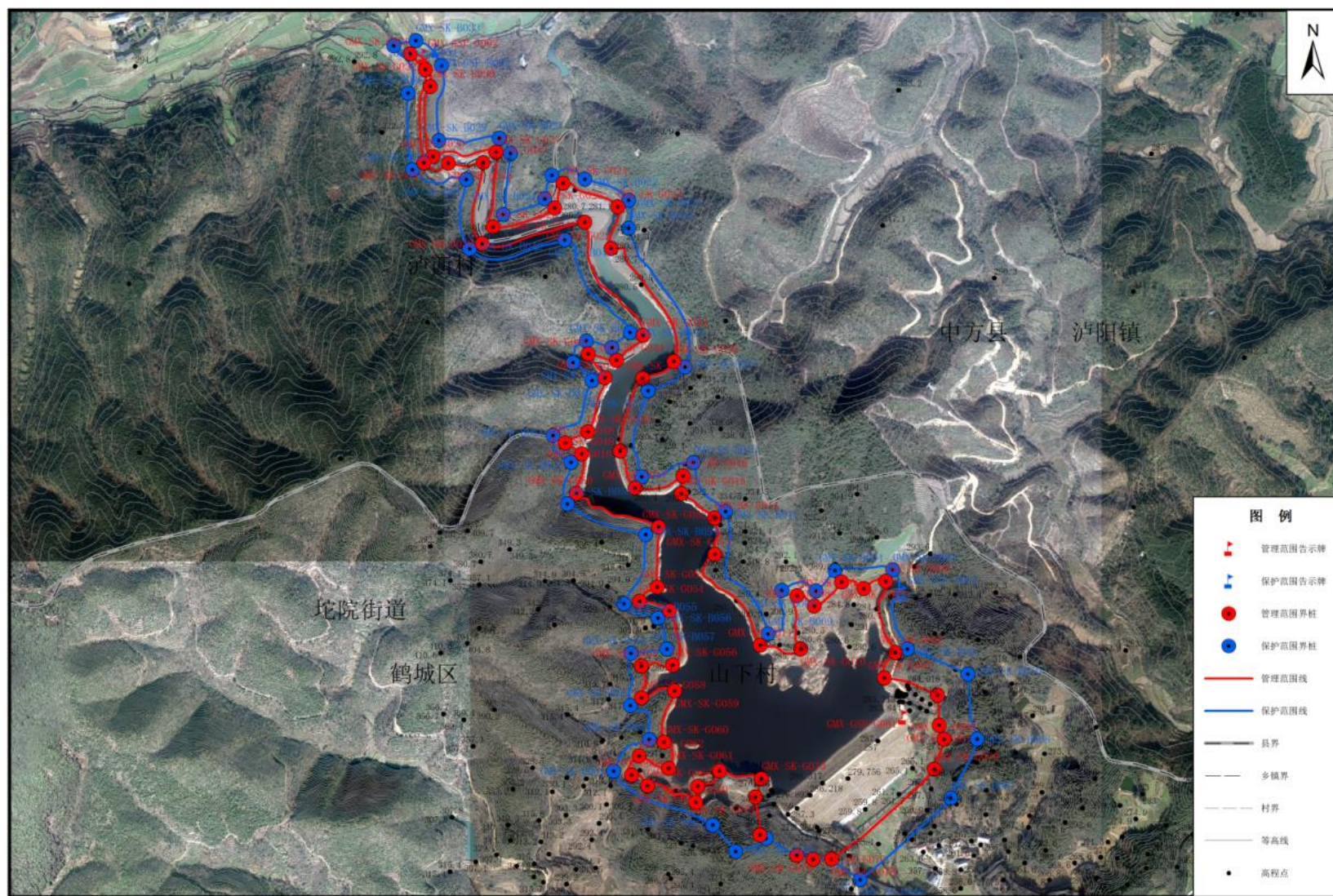
革命溪水库工程管理与保护范围划界示意图
