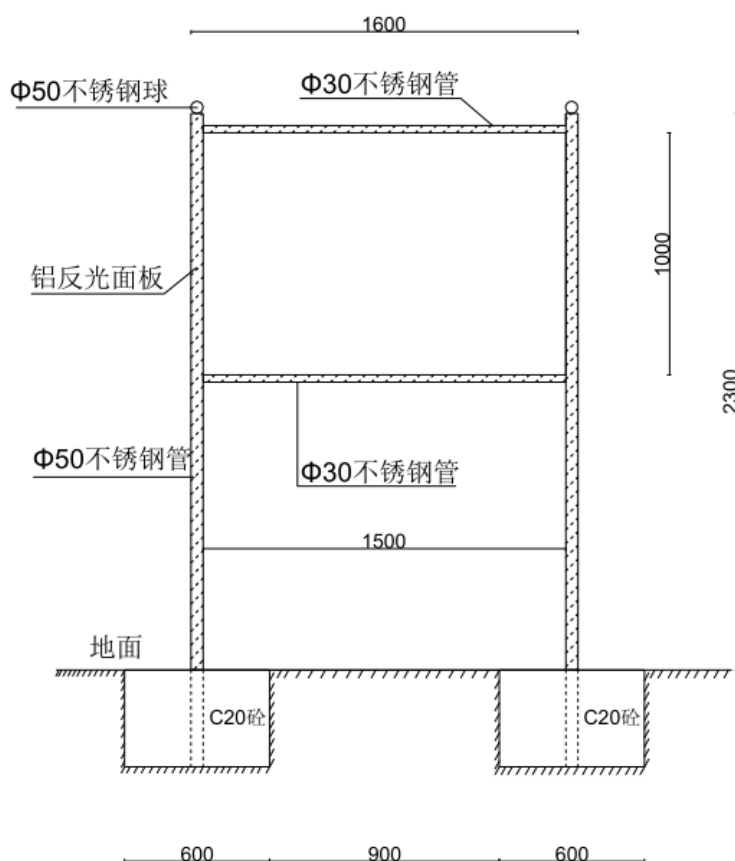
图 6.1-4 告示牌正面示意图
