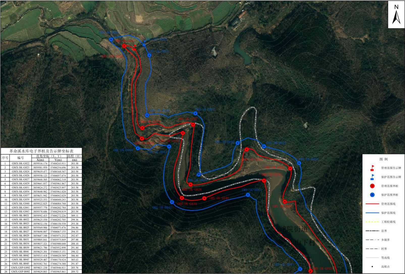
革命溪水库管理与保护范围划界图-004
