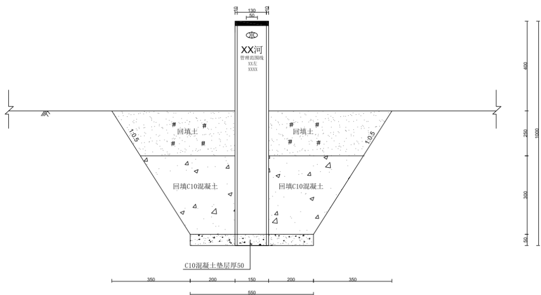
图 6.1-2 界桩结构图
