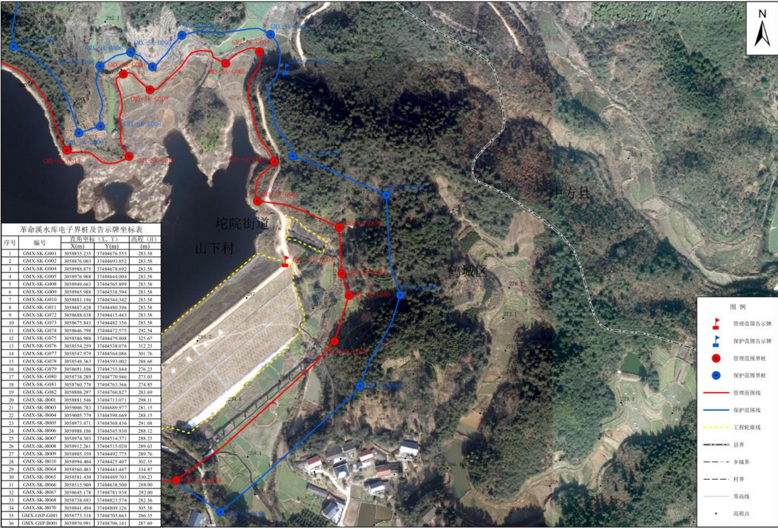
革命溪水库管理与保护范围划界图-001
