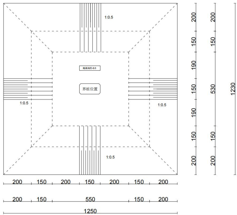
图 6.1-2 界桩结构图
