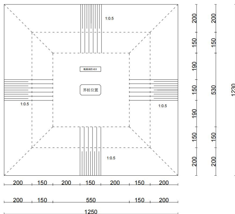
图 6.1-3 界桩平面图
