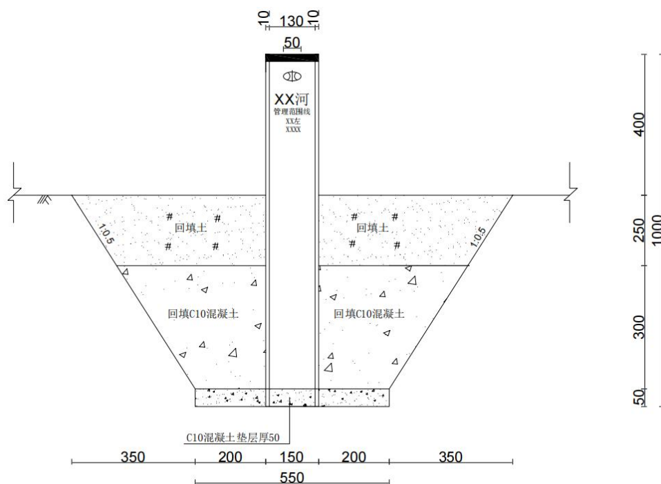
图 6.1-2 界桩结构图
