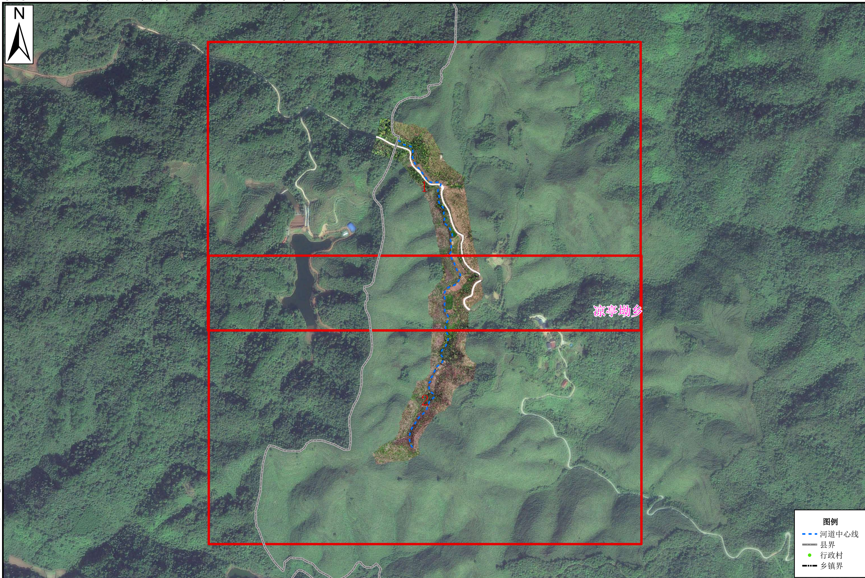
图二 甲岩溪鹤城区河段河道管理范围划定总图
