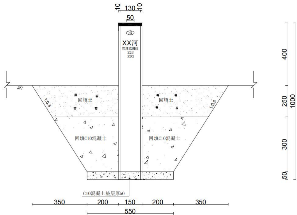
图 6.1-2 界桩结构图
