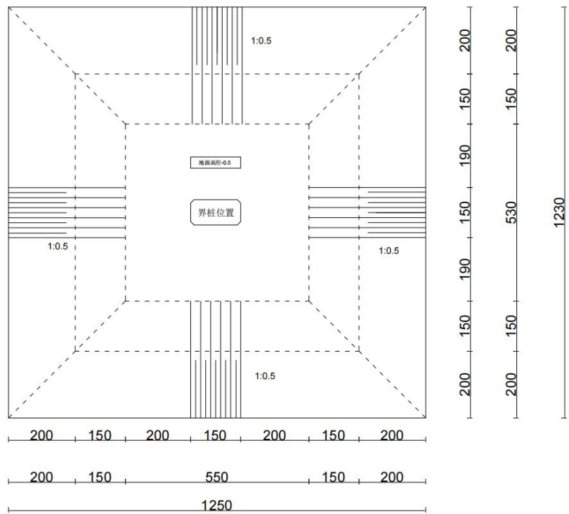
图 6.1-2 界桩结构图
