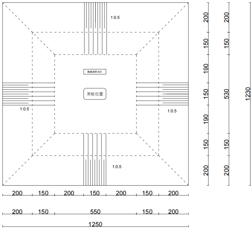
图 6.1-2 界桩结构图
