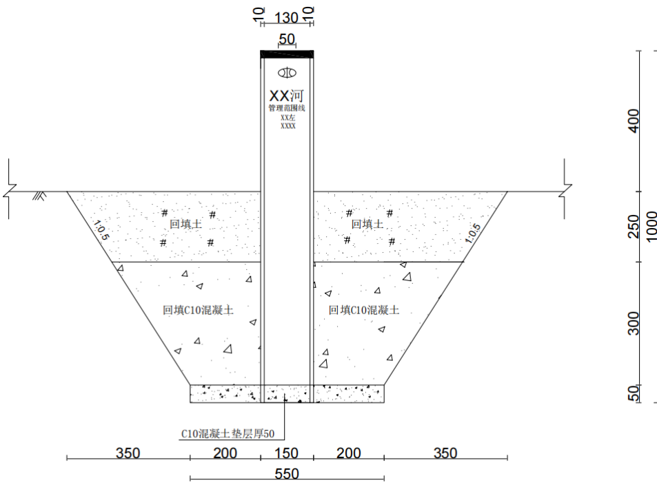
图 6.1-2 界桩结构图
