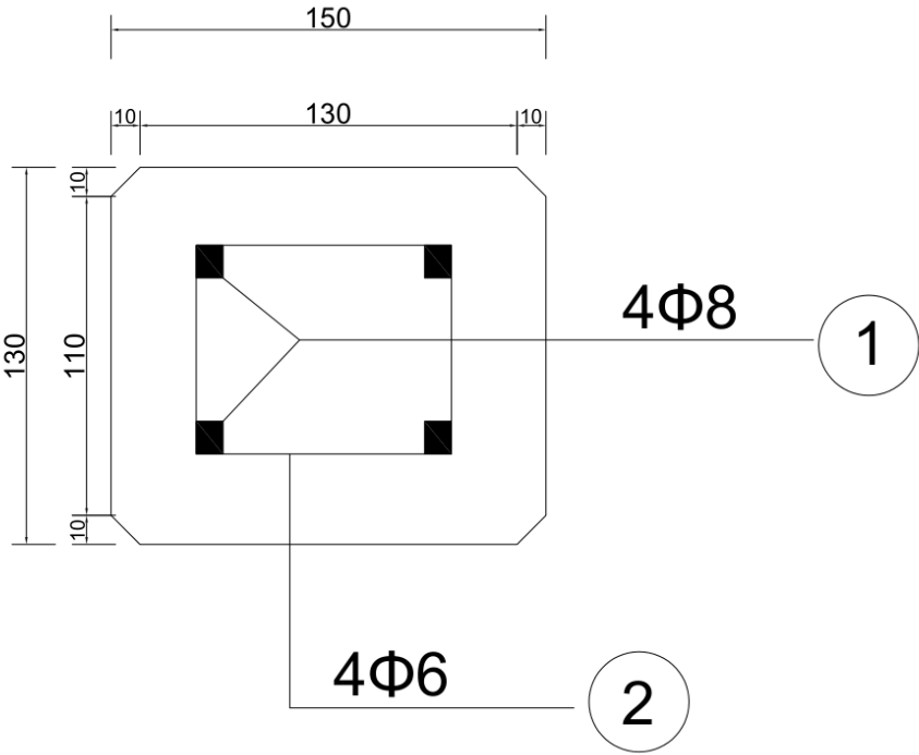
图 6.1-1 界桩钢筋配置图
