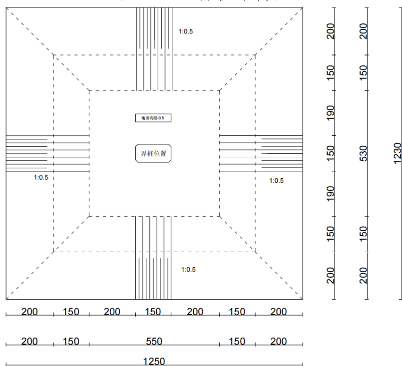
图 6.1-2 界桩结构图
