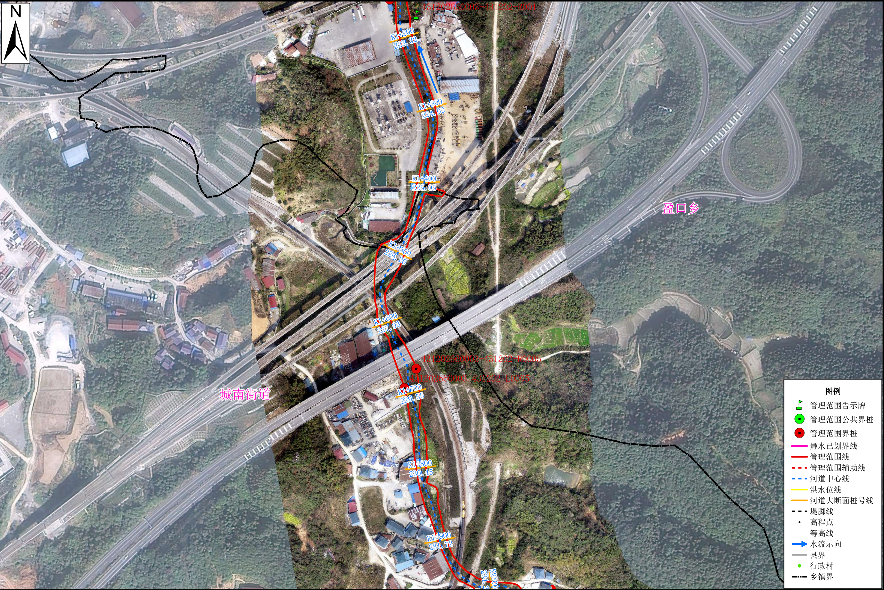
分图2 青山溪河道管理范围划定图（2/7）
