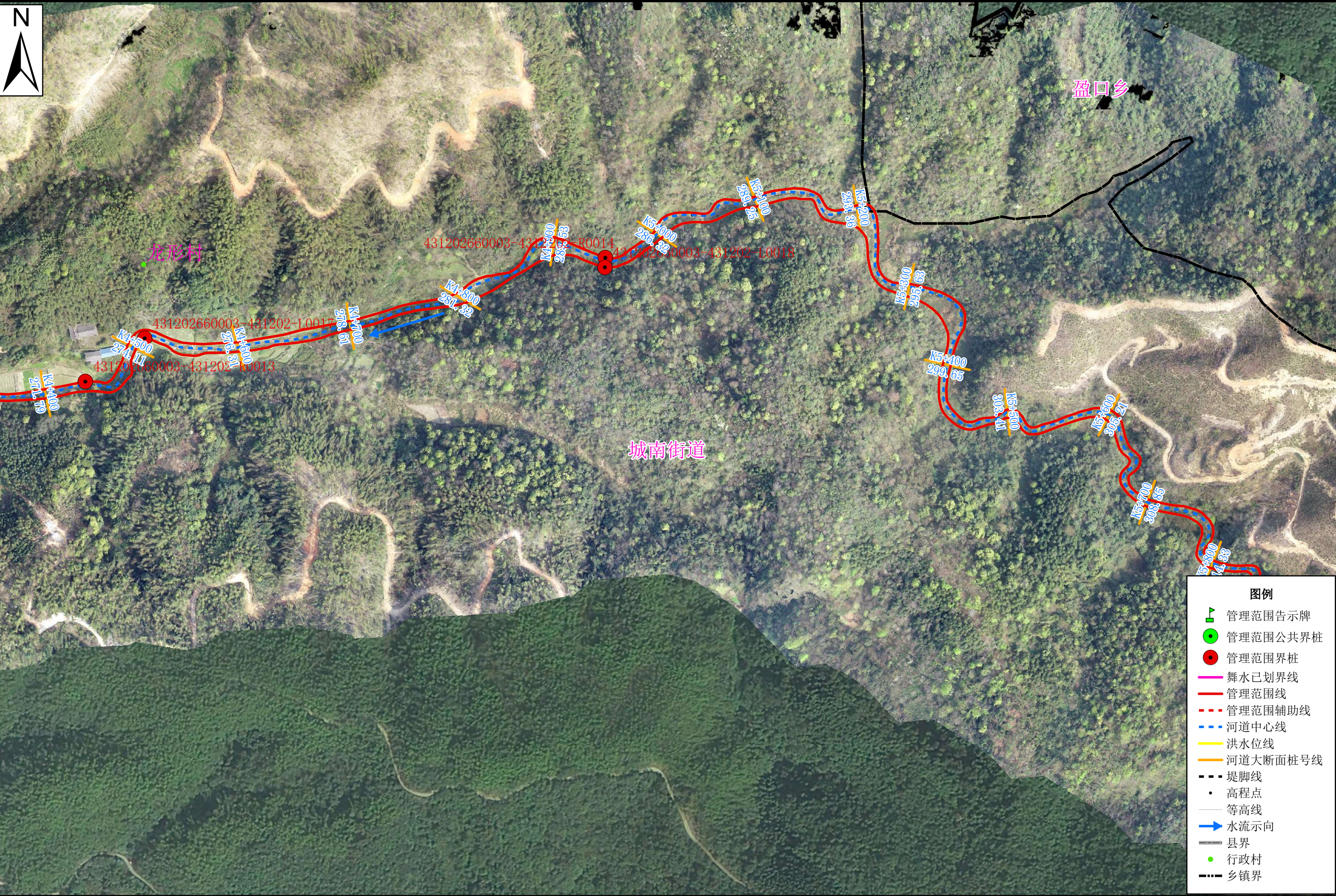
分图5 青山溪河道管理范围划定图（5/7）
