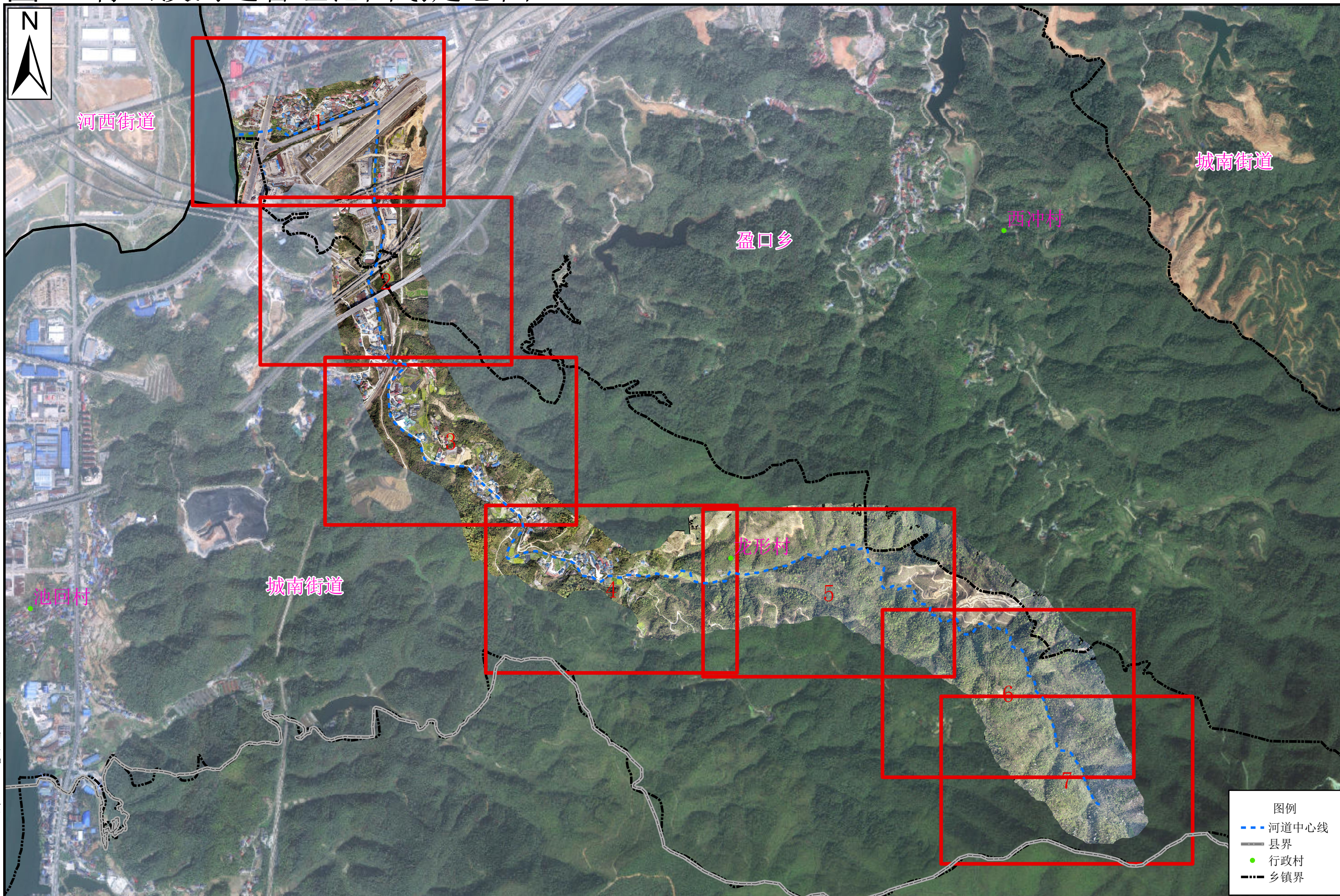
图二 青山溪河道管理范围划定总图
