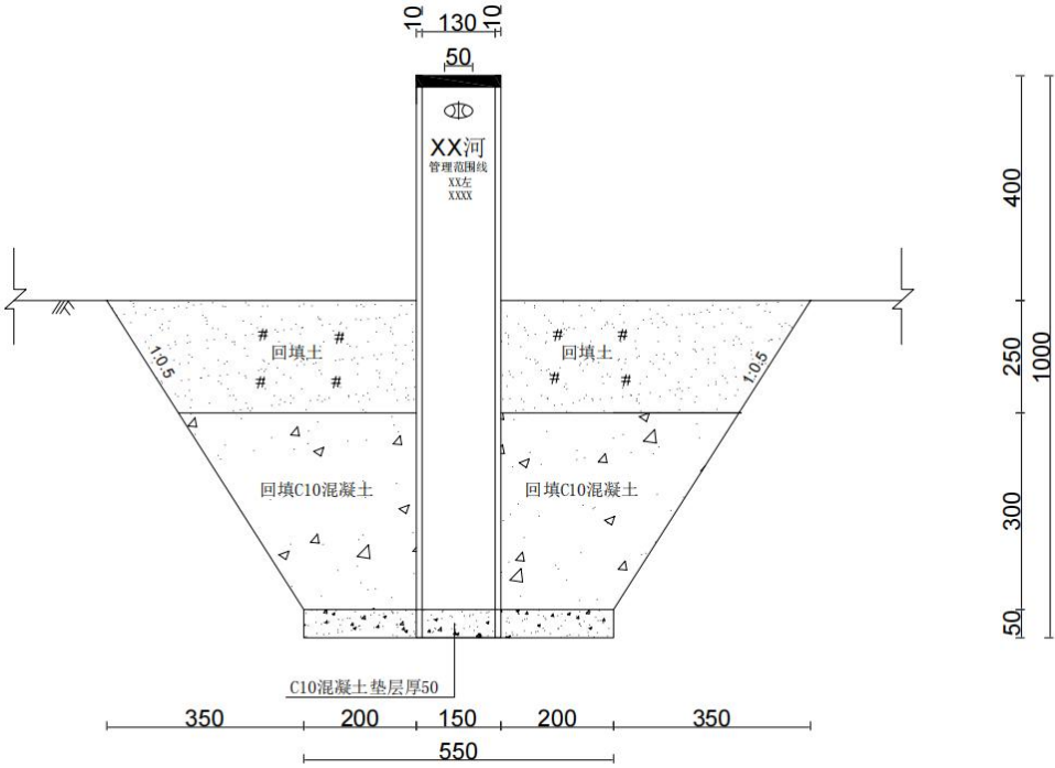
图 6.1-2 界桩结构图
