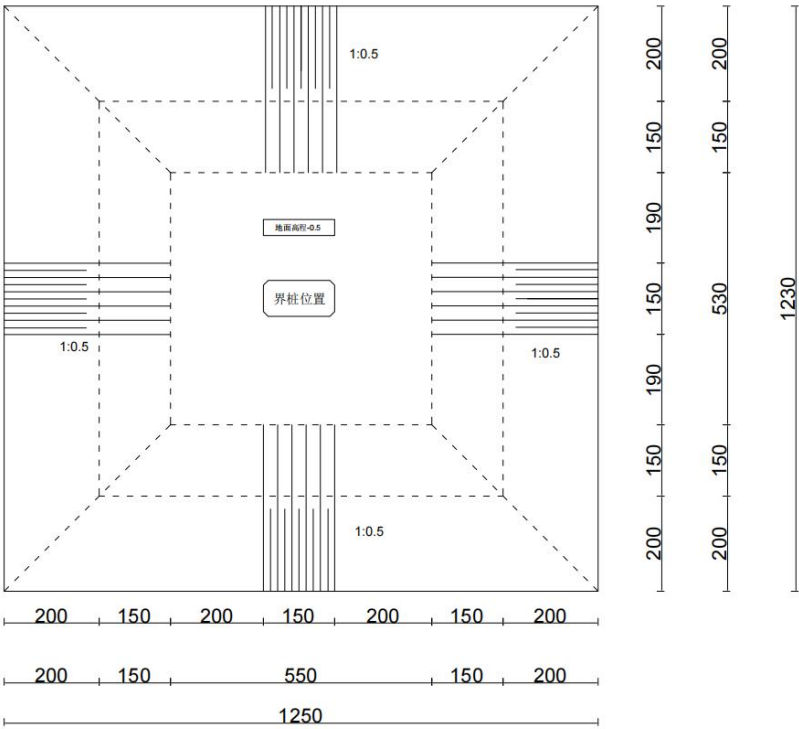
图 6.1-2 界桩结构图
