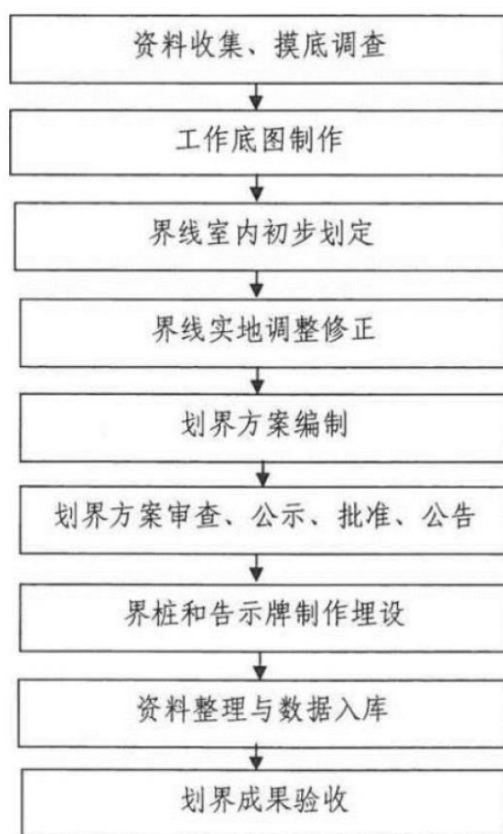
图 4.1-1 河道管理范围划界总体工作流程图
