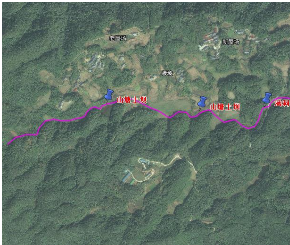
图 2.3-1 烂溪口溪涉河建筑物示意图
