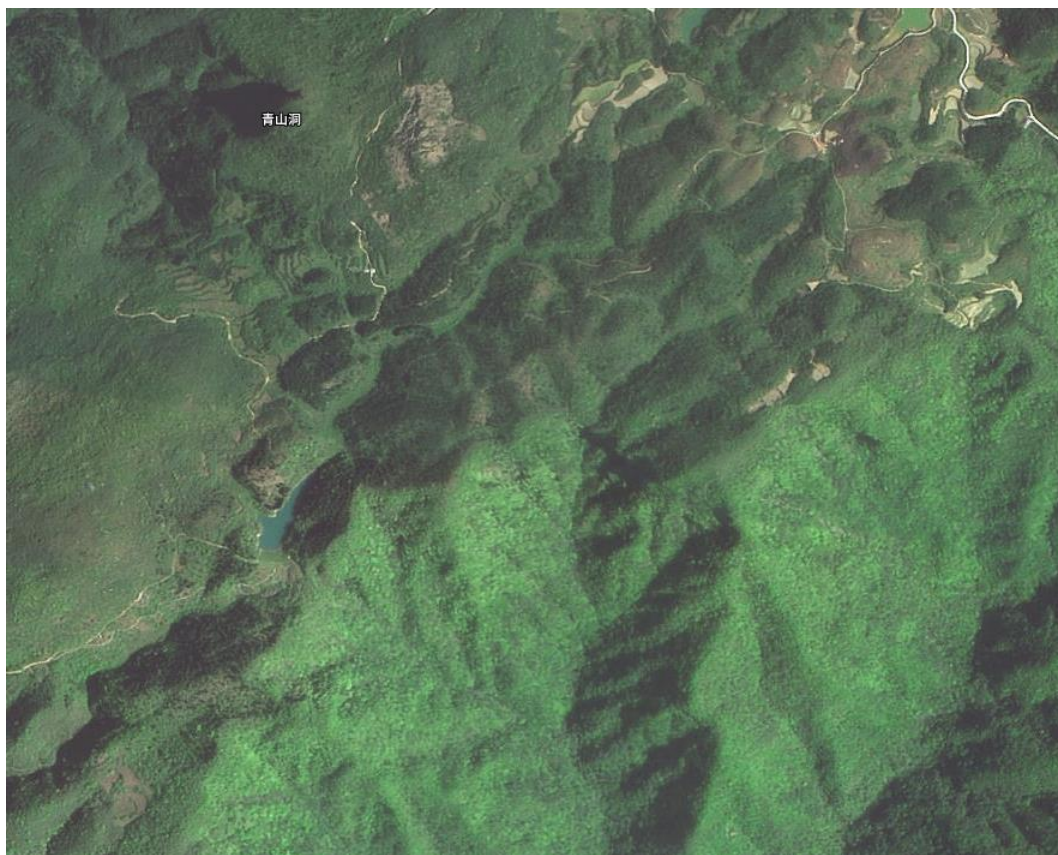
图 1.1-3 坨院溪河源位置图
