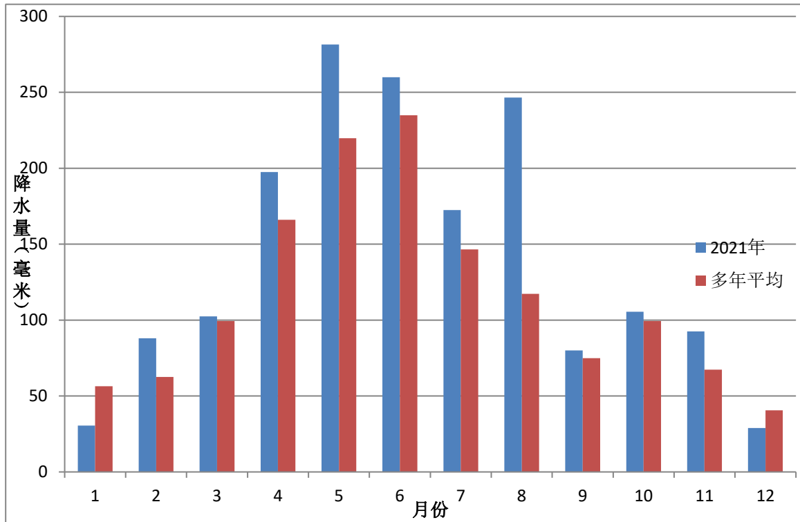
图 1.1-12 怀化市降水分配图
